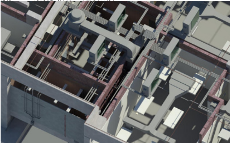
BIM模型（建筑信息模型）：可模拟和描述网络、结构、建筑具体构造的模型
